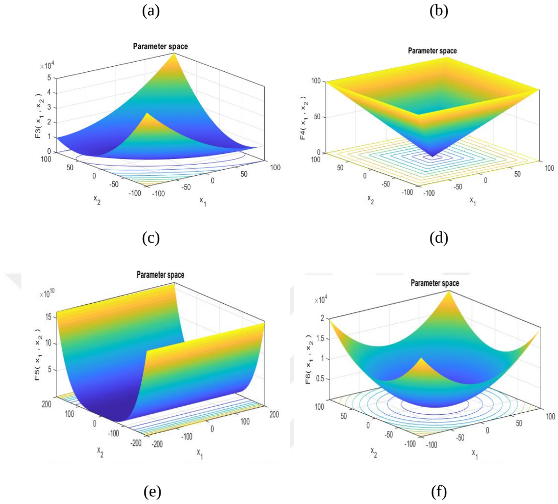
Figure 3.9: Benchmark Functions, (a) F_1 Function Parameter Space, (b) F_2 Function Parameter Space, (c) F_3 Function Parameter Space, (d) F_4 function Parameter Space, (e) F_5 Function Parameter Space, (f) F_6 Function Parameter Space
