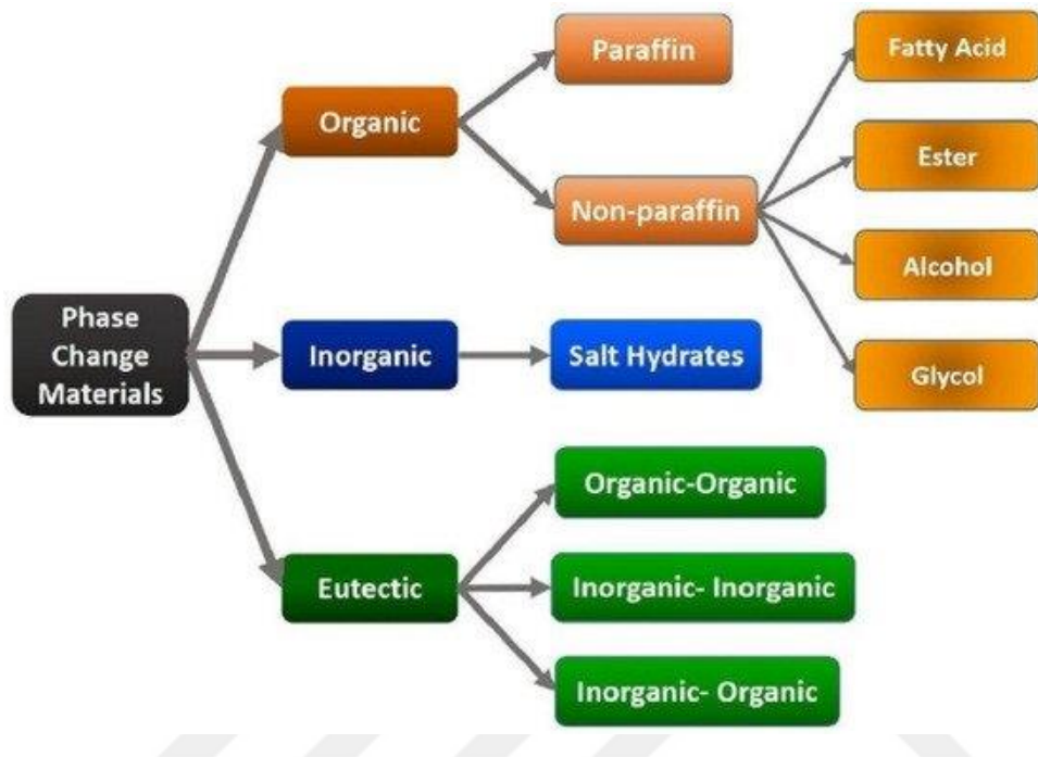
Figure 2.1 PCM Categorization (Barbi, Barbieri, Marinelli, Rimini, Merchiori, Bottarelli & Montorsi, 2022)
