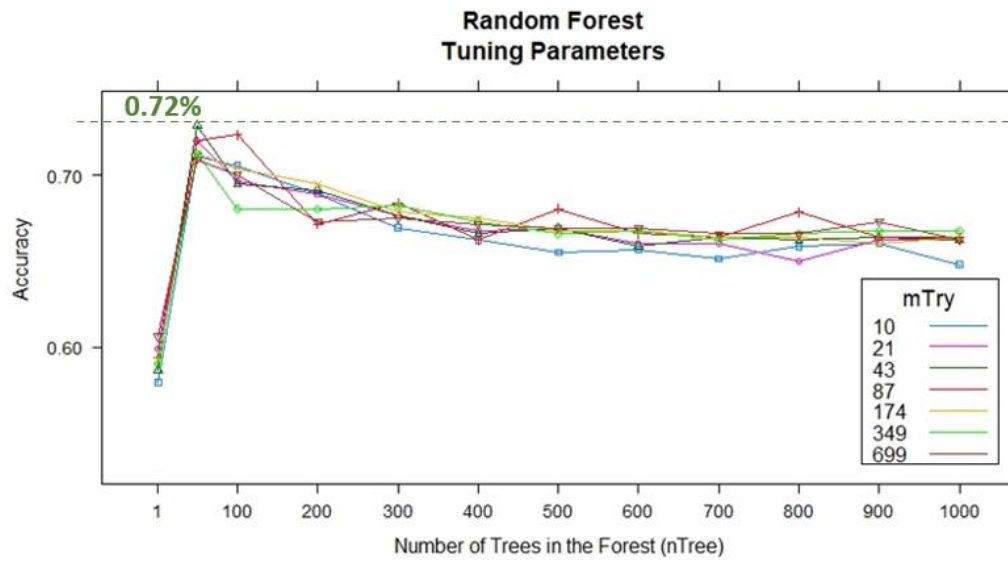
Figure 19: ADNI RF Tuning Parameters
