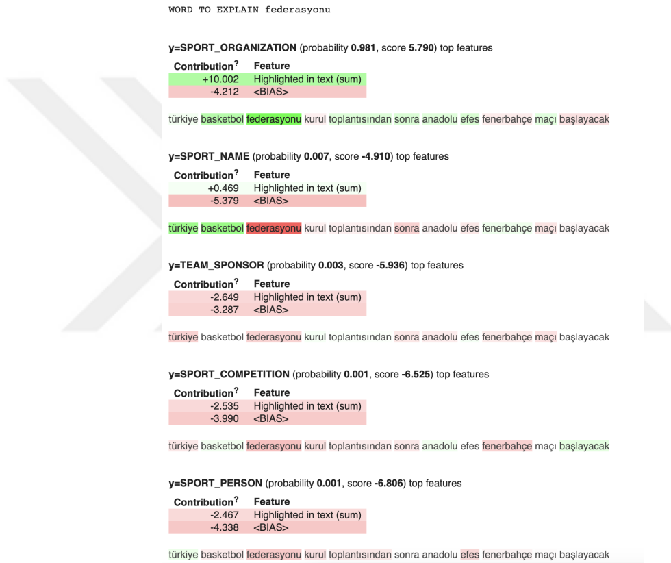
Figure 4.23: Explanation of the word federasyonu in the sentence türkiye basketball federasyonu kurul toplantısından sonra anadolu efes fenerbahçe maçı başlayacak by LIME.
