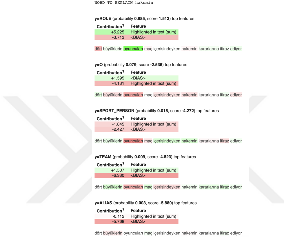
Figure 4.25: Explanation of the word hakemin in the sentence dört büyüklerin oyuncularını maç içerisindeyken hakemin kararlarına itiraz ediyor. by LIME.
